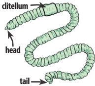
FIG. 25: Earthworm body plan
